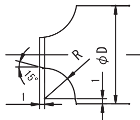
刃先形状
